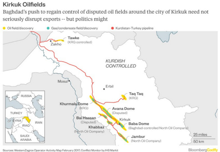
Grafik 1: Kuzey Irak'taki petrol & doğalgaz sahaları ve boru hatları
